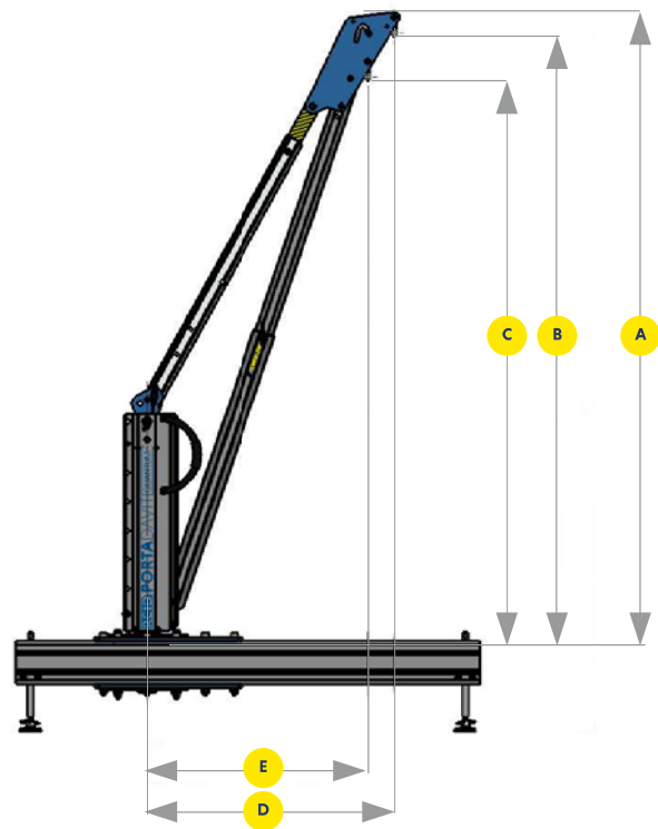
DIMENSIONES (MM)
