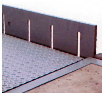
Rampa en reposo con el labio de seguridad dispuesto.
