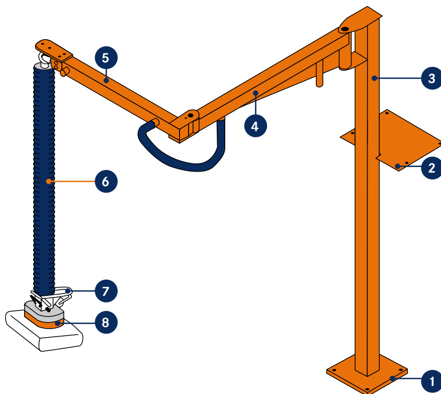
Pluma columna articulada.
